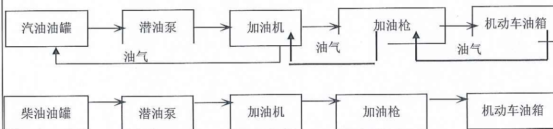
加油工艺流程图
